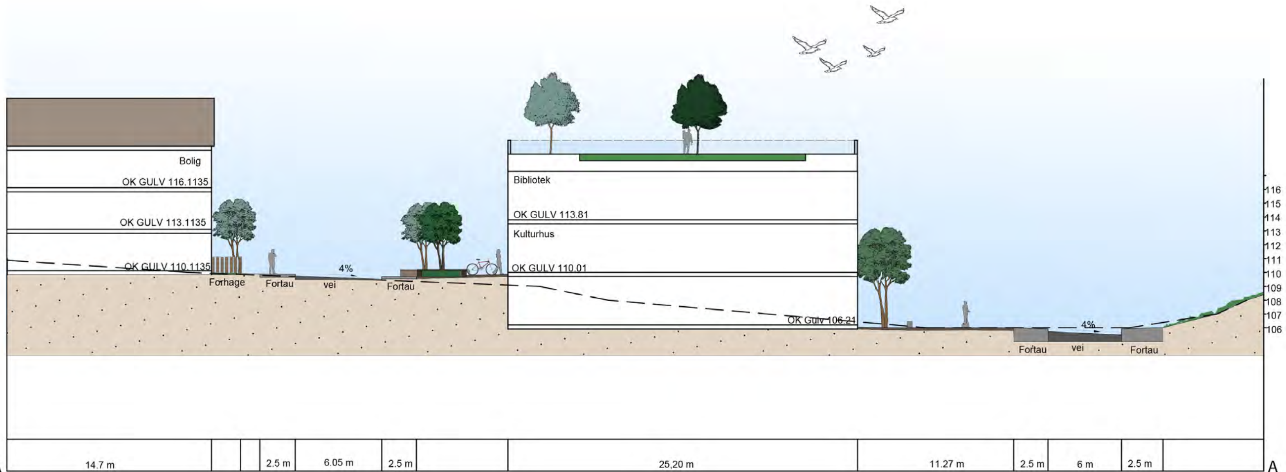
Oppriss - 1:300 fra Sør til Nord av Kulturhuset og tre etasjers bolig
